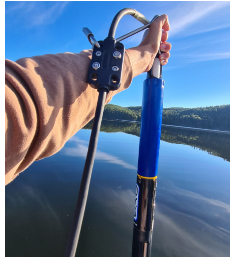
Sonde til bruk ved vertikalprofil av vannsøylen i innsjøer. Foto: Lisa Nielsen, Norconsult.
