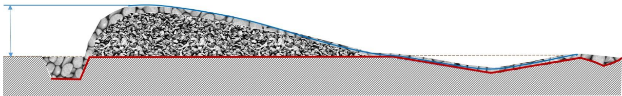
Figur 3. Snitt av permeabel terskel. Denne terskelen er mest aktuell, men terskeltype «hoppesteinterskel» kan også anlegges ett eller to steder.
