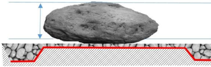
Figur 4: Hoppesteinterskel sett fra siden og ovenfra. Steinene kan gjerne presses litt ned i undergrunnen, og steinene som ligger ytterst presses inn i kanalsiden.
